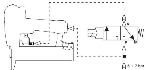
SZELEP 3/2 NC
