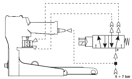
SZELEP 5/2
