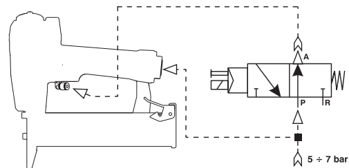
SZELEP 3/2 NO
